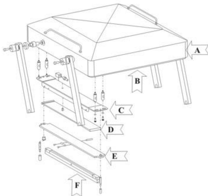
Рис 3 Деталировка изогнутой вакуумной крышки (для серии SC, SD).
